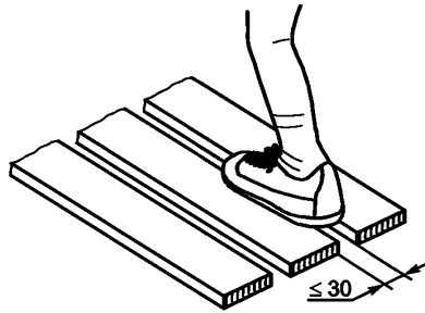
Рисунок 10 — Ширина зазоров на поверхностях наклоном до 45°
